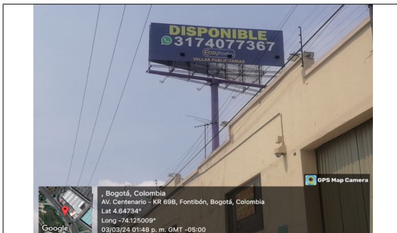
Fotografía No. 2 – Vista del panel y de la estructura tubular instalada concéntricamente.
